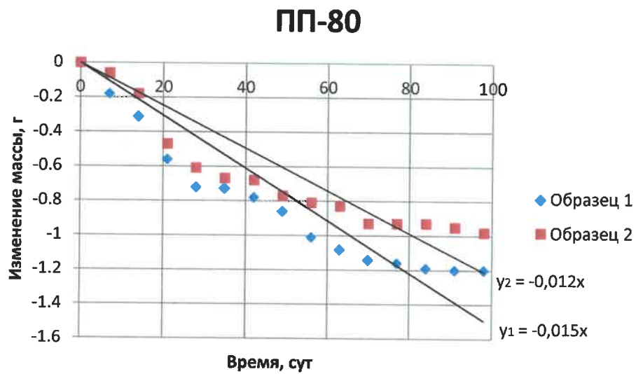
Рис. 4.7 Абсолютное изменение массы образцов ПП-80 в процессе испытаний
