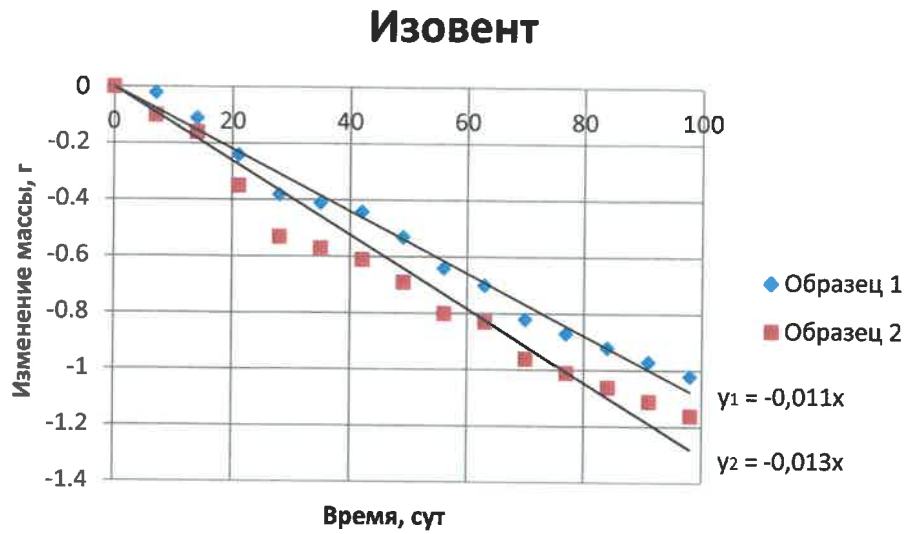
Рис. 4.6 Абсолютное изменение массы образцов Изовент в процессе испытаний
