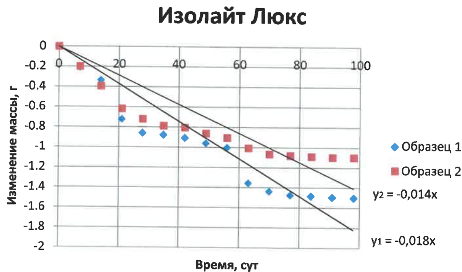
Рис. 4.5 Абсолютное изменение массы образцов Изолайт Люкс в процессе испытаний
