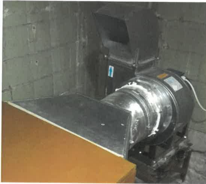
Рис. 3.2 Вентилятор, вмонтированный в экспериментальную установку
