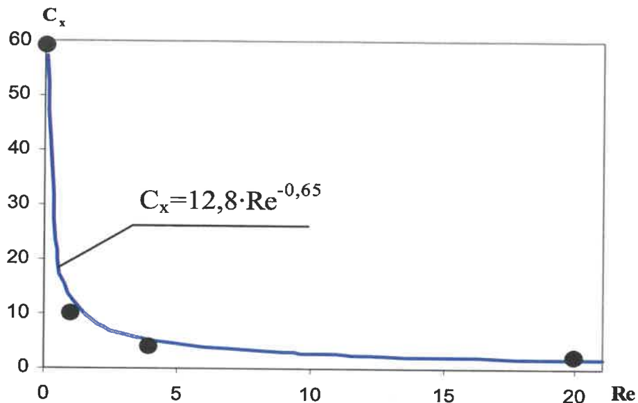
Рис. 2.1 Зависимость коэффициента сопротивления цилиндрического волокна от числа Рейнольдса [20] (точки – экспериментальные данные, кривая – степенная аппроксимация)
