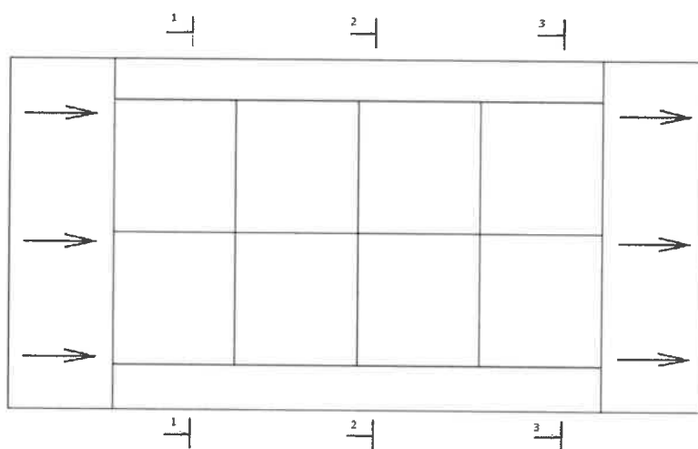
Рис. 3.1 Схема короба для экспериментальной установки для исследования эмиссии волокон из минераловатных плит
